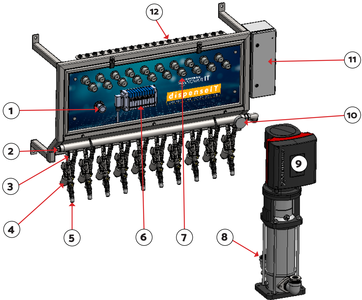
Fig. 2.1 - 1 - dispenseIT identification
